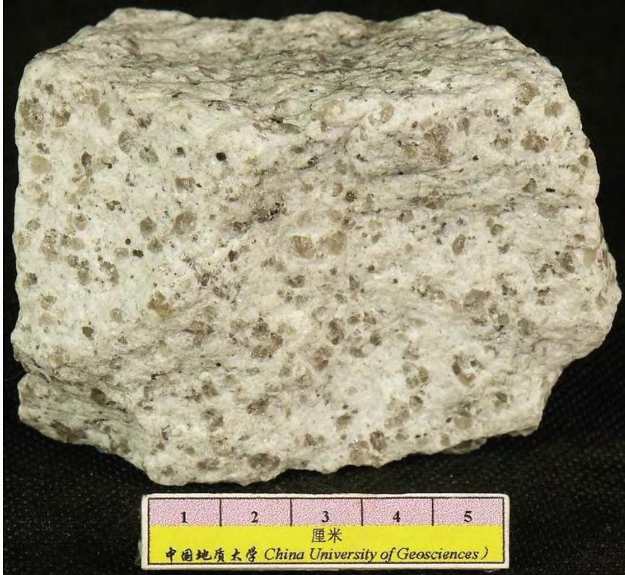
岩石名称：白岗岩 英文名称：Alaskite 颜色：浅灰白 构造：块状构造 结构：中晶结构 主要成分：长石、石英 所属岩类：岩浆岩\酸性深成侵入岩 产地：北京八达岭
