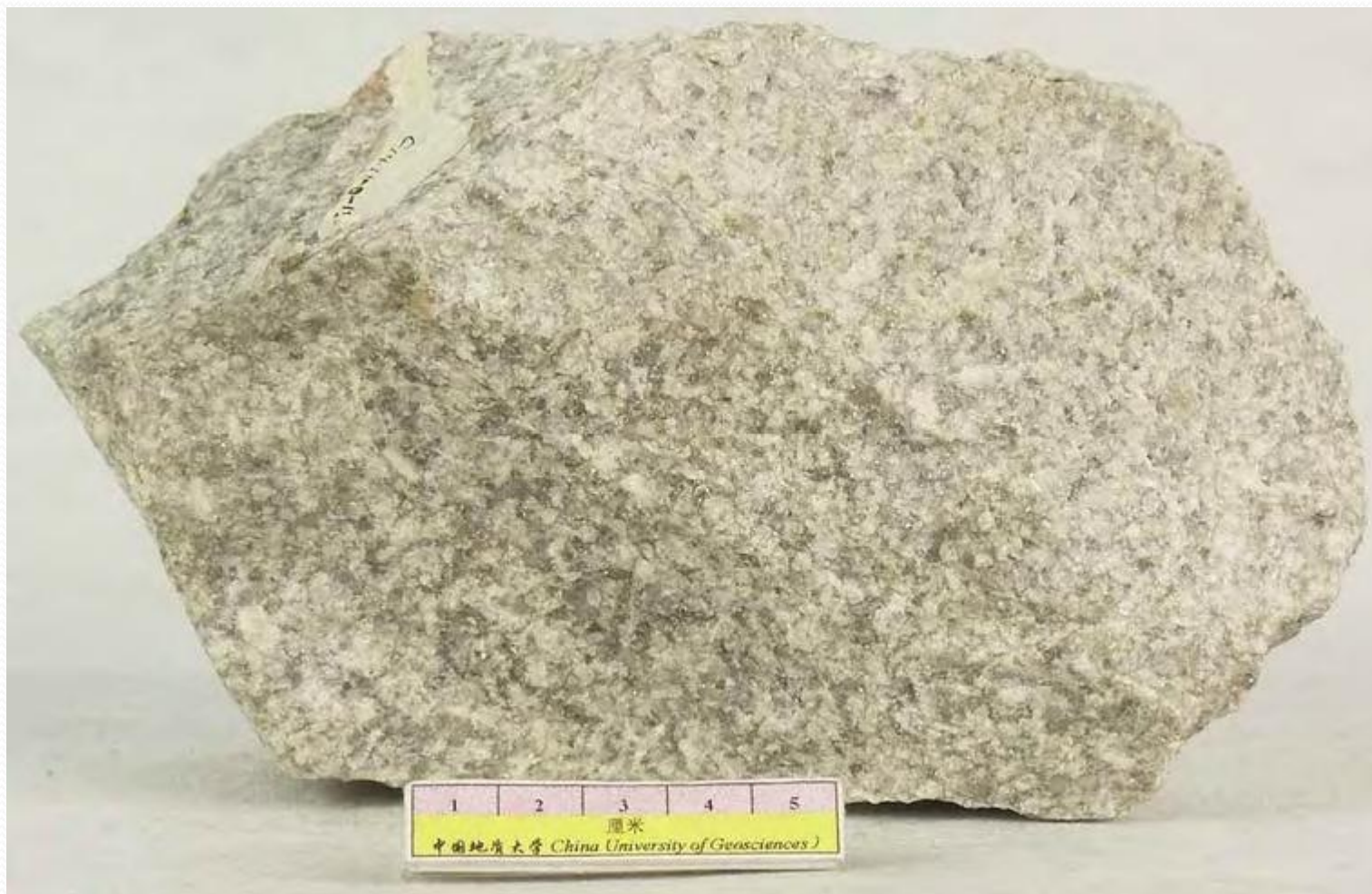
岩石名称：中细粒花岗岩 英文名称：Medium-fine granite 颜色：浅灰 构造：块状构造 结构：中细晶结构 主要成分：石英，钾长石 所属岩类：岩浆岩\酸性深成侵入岩 产地：江西宜春
